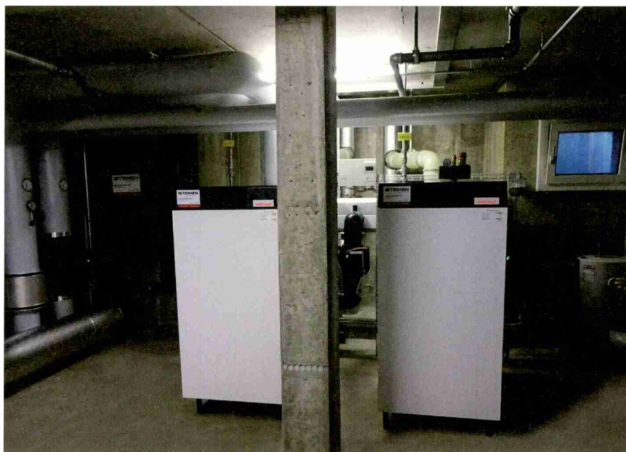
Die beiden Weishaupt Thermo Condens WTC-GB 300 Gas-Brennwertkessel in der Bärenweid-Zentrale.
